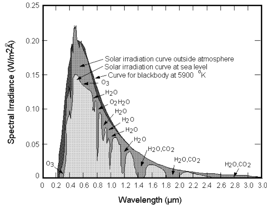
Fig. Spettro di emissione del sole al di fuori dell'atmosfera confrontato con l'emissione di un corpo nero con T=5900\text{K} (in chiaro lo spettro misurato al livello del mare con gli assorbimenti dovuti alle molecole presenti nell'atmosfera)
